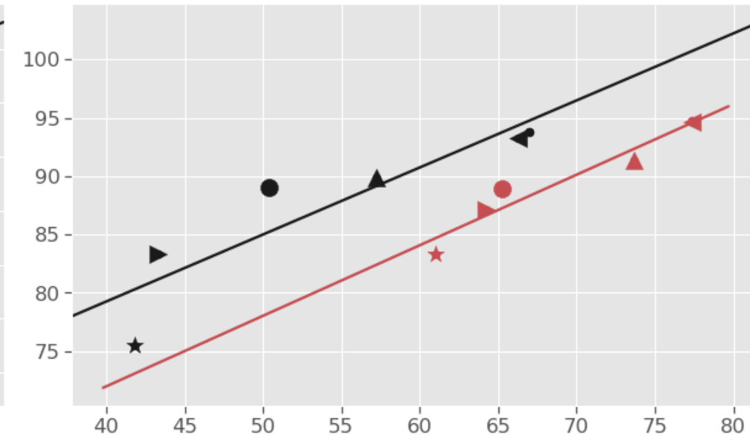
Caltech-101
