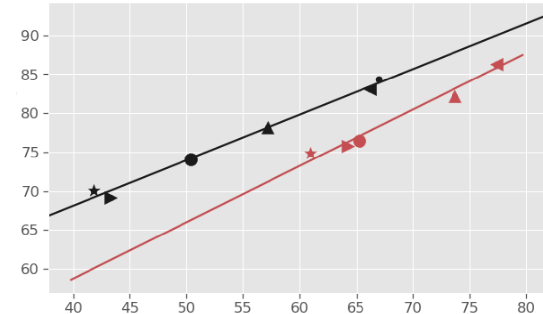
Caltech-256
